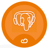
a9s PostgreSQL
